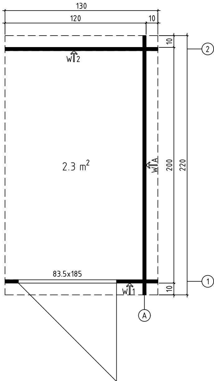
GROUNDPLAN - GRUNDPLAN - PLAN DE MASSE
